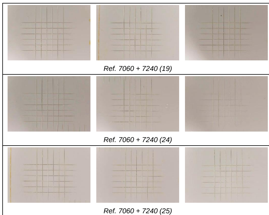
Figura 6. Aspecto de las muestras tras el ensayo de adherencia por corte enrejado tras 480 horas de niebla salina
